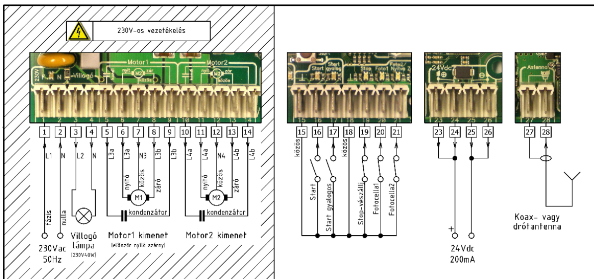
Sorcsatlakozók bekötése
